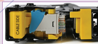
Salida/Outlet Híbrido
